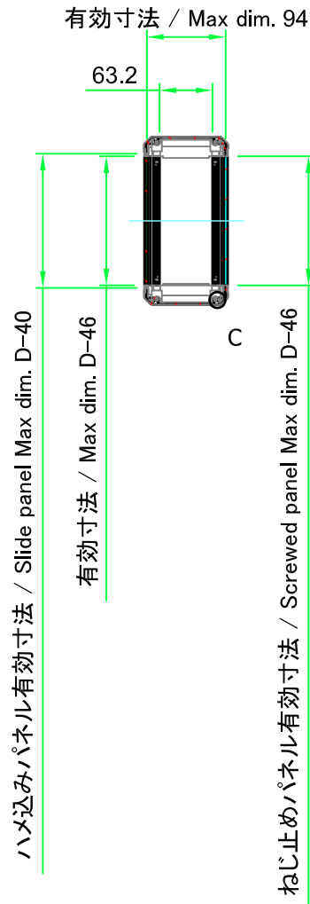
C : フレーム拡大図 Frame cross-section
